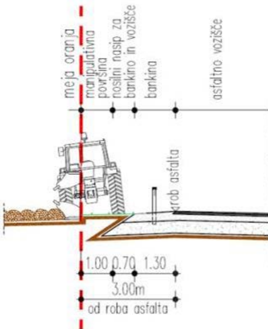
Slika 1 – ORANJE VZPOREDNO S CESTO
