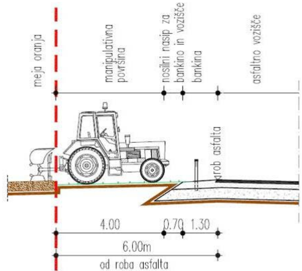
Slika 3 - ORANJE PRAVOKOTNO NA CESTO
